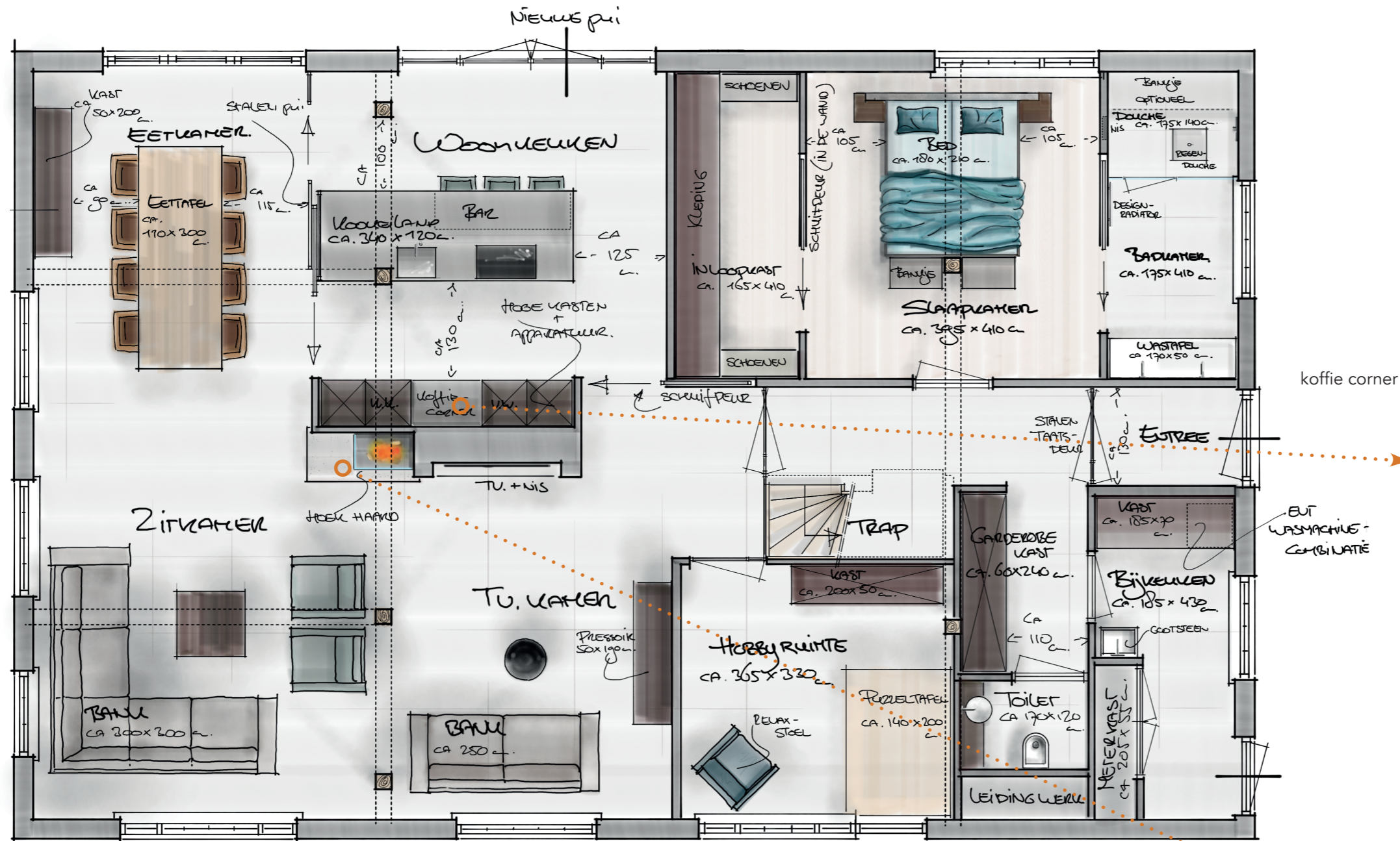
Plattegrond begane grond: geen schaal
